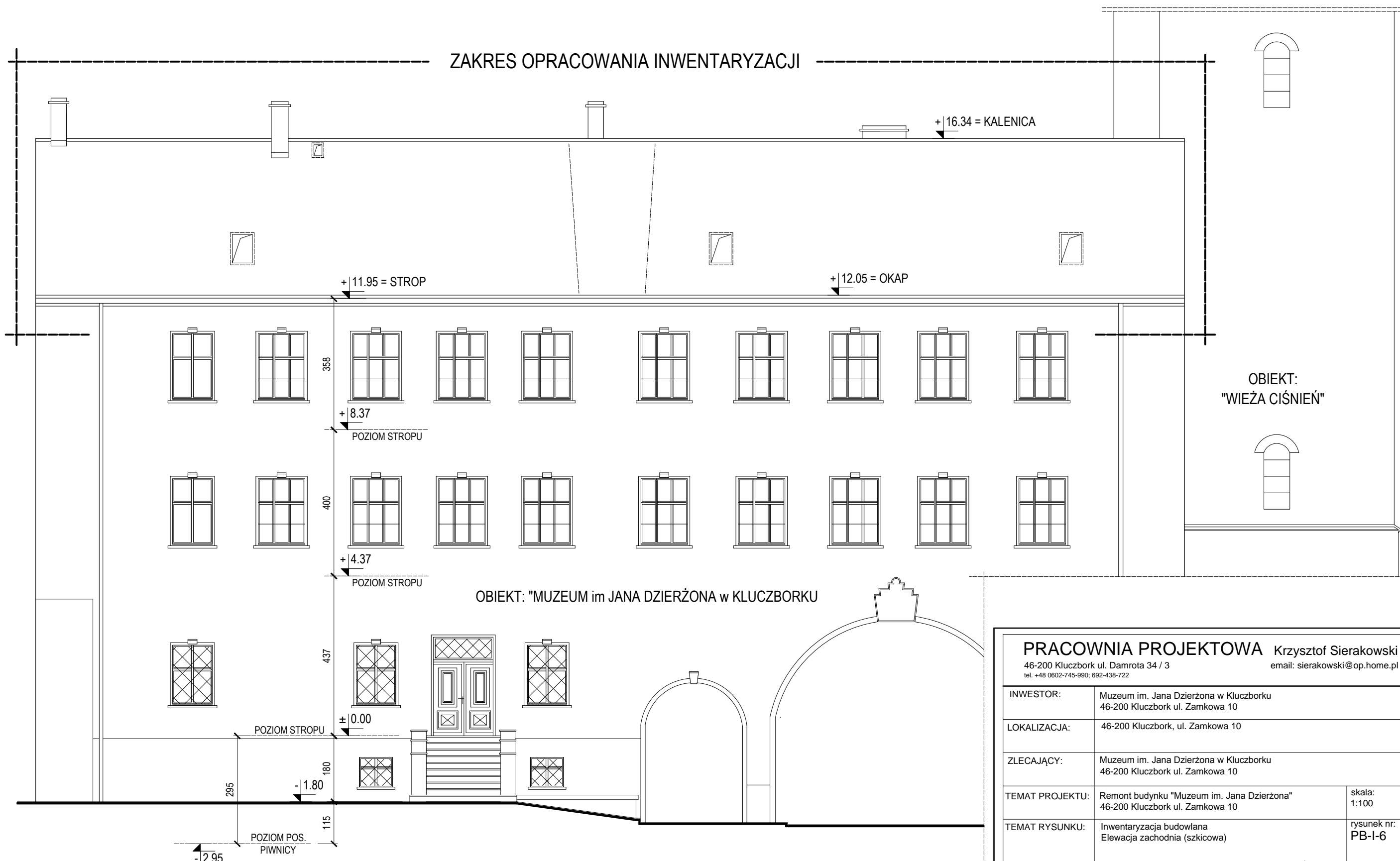
INWENTARYZACJA BUDOWLANA - ELEWACJA ZACHODNIA (SZKICOWA) skala 1:100
