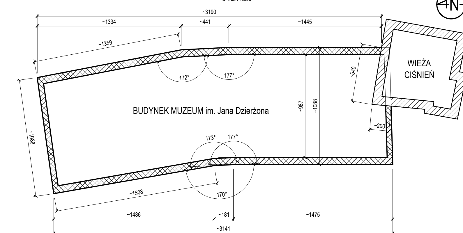
SKZIC BUDYNKU - UKŁAD ŚCIAN ZEWNĘTRZNYCH - POZIOM STRYCHU SKALA 1:200
